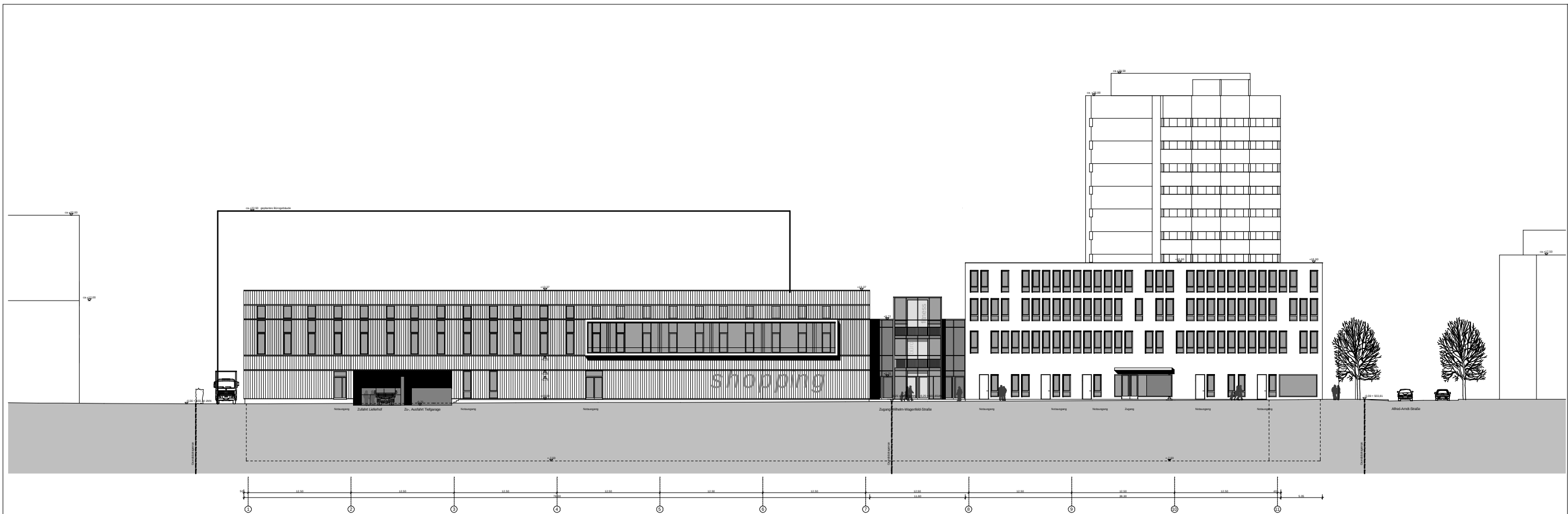
ansicht süd
