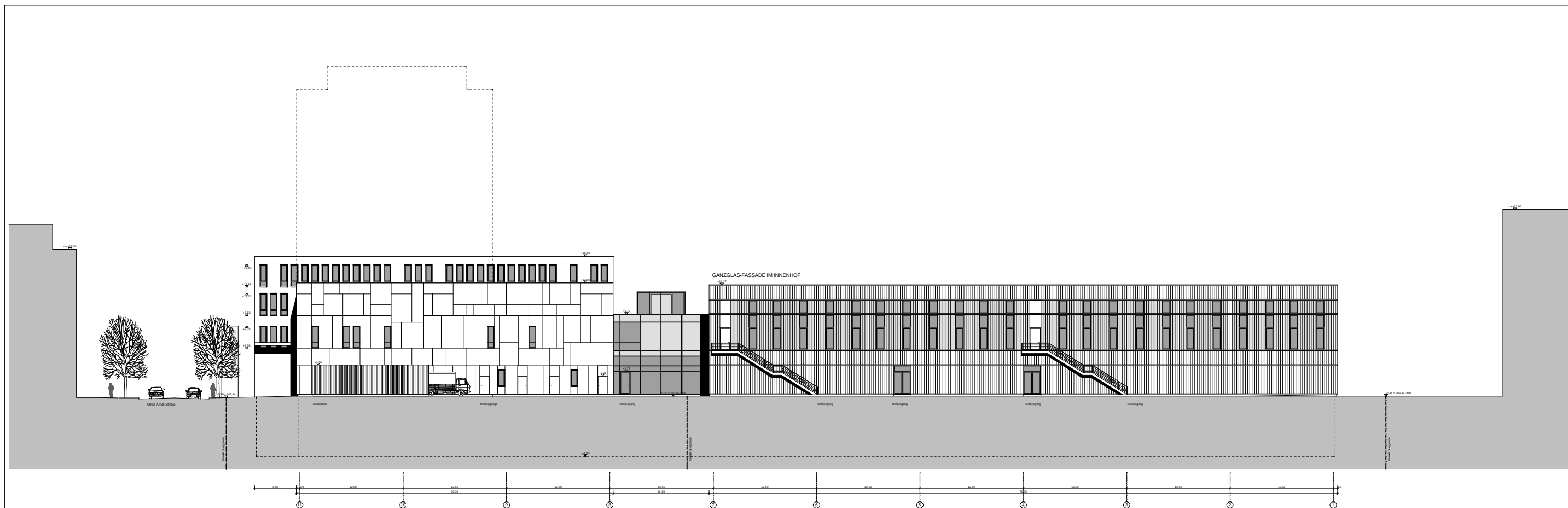
ansicht nord
